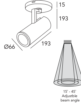
S-T-203/xx-COB-23W-xK
