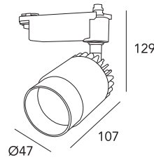
T-206/xx-COB-5W-xK
