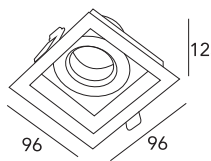
A-SQ-104/xx-MR16
