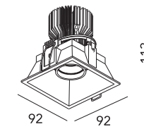
A-SQ-107/xx-MR16
