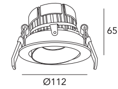
R-A-218/xx-COB-12W-3K
