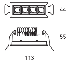
R-SQ-204/xx-COB-10W-3K
